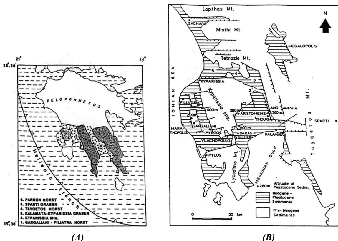
Εικ. 1. Οι 1 ης (Α) και 2 ης (Β) τάξης νεοτεκτονικές μακροδομές της ΝΔ Πελοποννήσου. Οι 2 ης τάξης νεοτεκτονικές μακροδομές του 1 ης τάξης τεκτονικού βυθίσματος Καλαμάτας-Κυπαρισσίας. 1: Τεκτ. βυθ. Κάτω Μεσσηνίας, 2: Τεκτονικός κέρας Μελιγαλά, 3: Τεκτ. βυθ. 'Ανω Μεσσηνίας, 4: Λεκάνη Δώριου, 5: Τεκτ. βυθ. Κυπαρισσίας-Καλού Νερού
